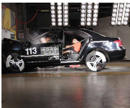
Collision frontale contre une barrière fixe
