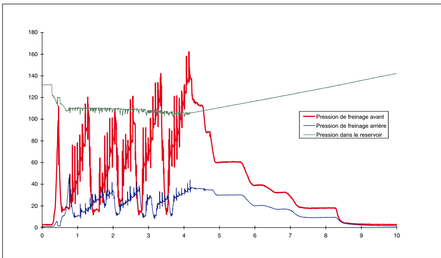
Développement de la pression de freinage d'une Ferrari après un freinage d'urgence avec système d'antiblocage
