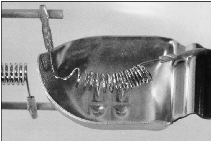
Ampoule de phare de moto après collision avec un piéton
