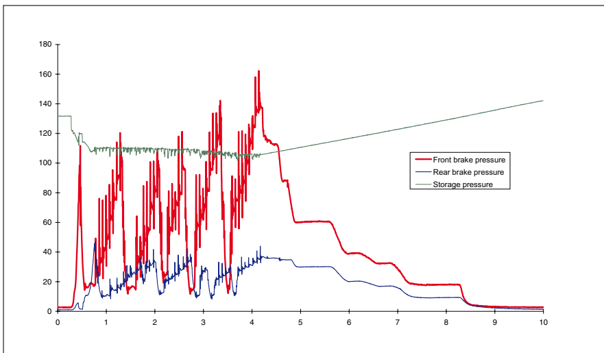
Brake pressure at a Ferrari after slamming on the brakes with ALS
